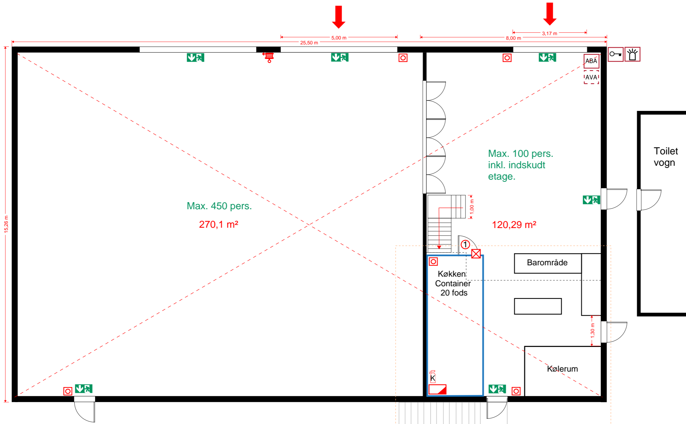
Indskudt etage
